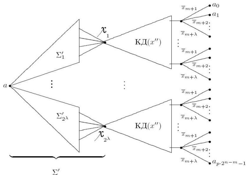
Рис. 7.1: к доказательству леммы 7.4
