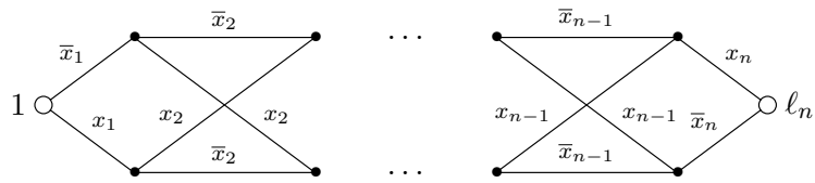
Рис. 3.4: схема Кардо для линейной функции l_n
