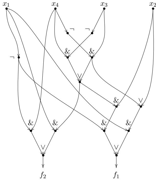
Рис. 3.3: СФЭ для системы ФАЛ F , построенная методом каскадов
