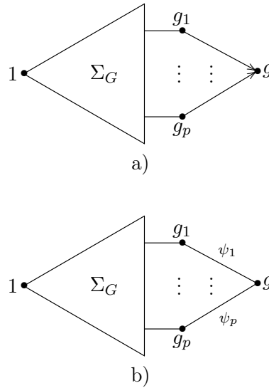
Рис. 6.1: Корректная реализация дизъюнкции ФАЛ g_1, \dots, g_p в классах КВС и ИКС
