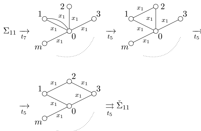
Рис. 7.7: вывод t_{11}
