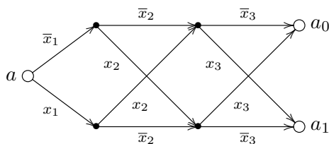
Рис. 10.4: BDD для l_3
